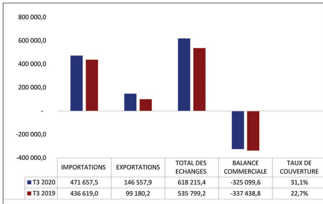
Graphique 1 : Les indicateurs du commerce extérieur du Burundi au 3 ème trimestre 2020 versus 2019
